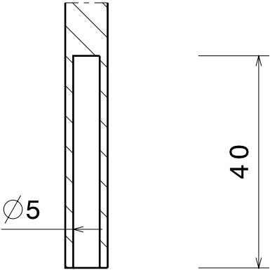
Plan Scale 1:1 Section A-A
